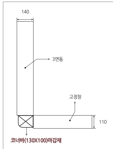
3연동 ㄱ자 중문 단면도
