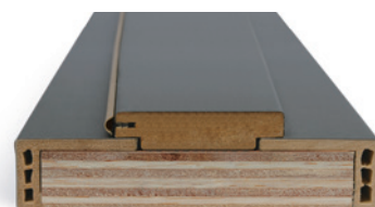
문선 없는 형 (가틀캡 50×30)
