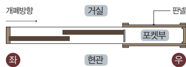
좌측개구설치(반대방향)
