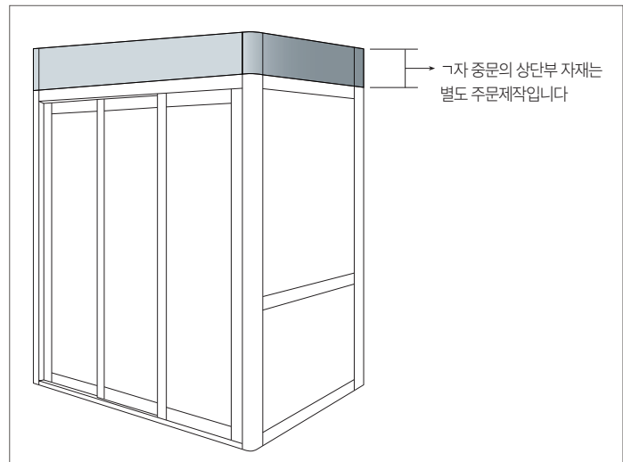
3연동 ㄱ자 중문 상부는 시공 시 설치
