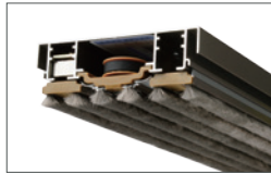
댐퍼 3연동 상부 철물
