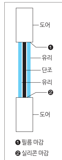
유리 접합 방식 (209F, 211F)
