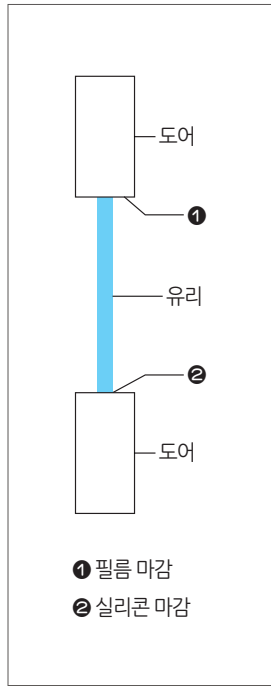
유리 접합 방식 (209, 211, 212, 290, 291)
