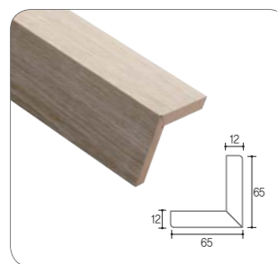
코너65 | 65×65×12
