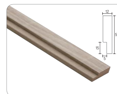
2계단 50 | 50×12
