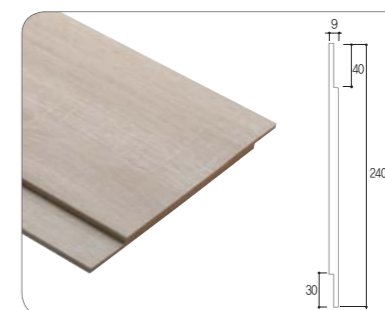
루버240 | 240×9
