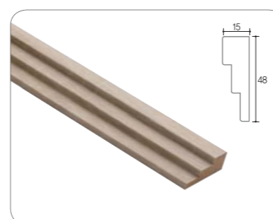
3계단 48 | 48×15
