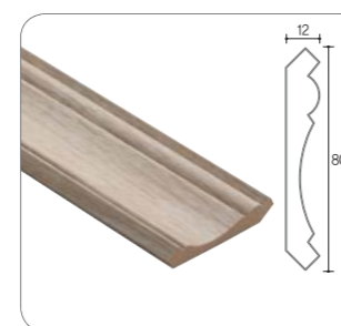
천정80 | 80×12
