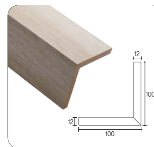
코너100 | 100×100×12
