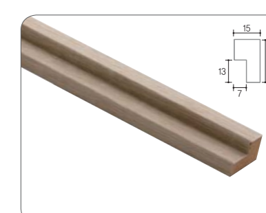
마이너스 | 25×15
