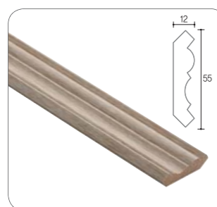
천정55 | 55×12
