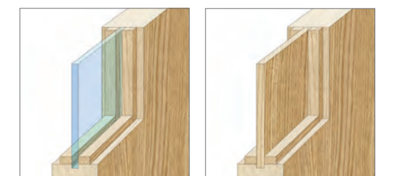
| 단면도 - 마감몰딩 매립형 (유리) | 단면도 - 마감몰딩 매립형 (고시)
