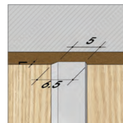
| NC가공상세도 [멤브레인패널] + 음각실크인쇄
