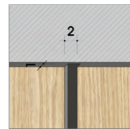
| NC가공상세도 [ABS패널]
