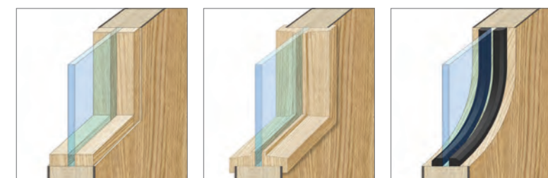
| 단면도 - 마감몰딩 매립형 | 단면도 - 마감몰딩 돌출형 | 단면도 - 마감몰딩 라운드형
