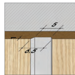
NC가공단면도 [멤브레인패널] + 음각 실크 인쇄
