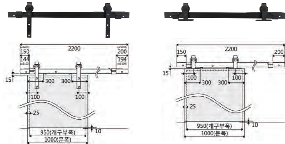
| 노출형행거도어1 HDLM-W3000D 도어전면 고정방식
